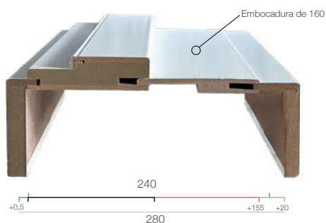
ALA 10 + C.BATEX 100 + EMBOCADURA 160 + ALA 25
