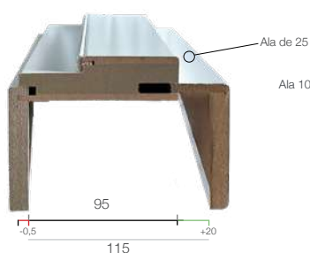
TADAP + C.BATEX 100 + ALA 25
