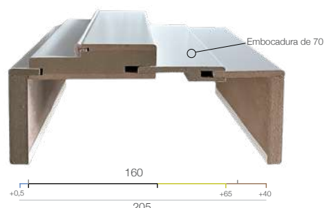
ALA 10 + C.BATEX 100 + EMBOCADURA 70 + ALA 45
