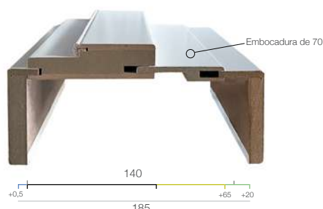
ALA 10 + C.BATEX 100 + EMBOCADURA 70 + ALA 25
