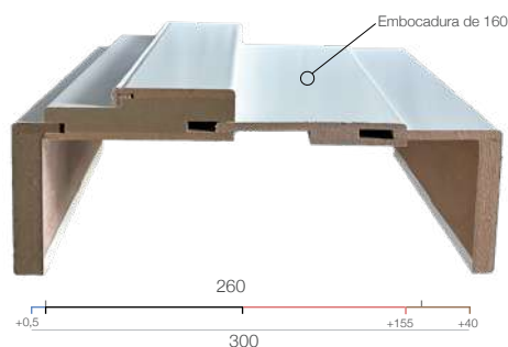
ALA 10 + C.BATEX 100 + EMBOCADURA 160 + ALA 45
