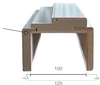
ALA 10 + C.BATEX 100 + ALA 25
